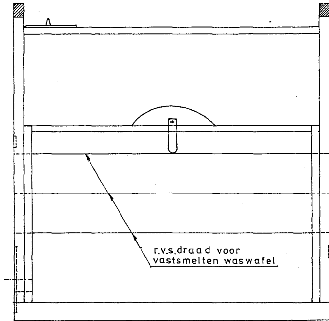
ZIJAAANZICHT
